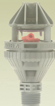
R2000LP/WF 0,9 a 5,7 GPM 191 a 1295 l/h
